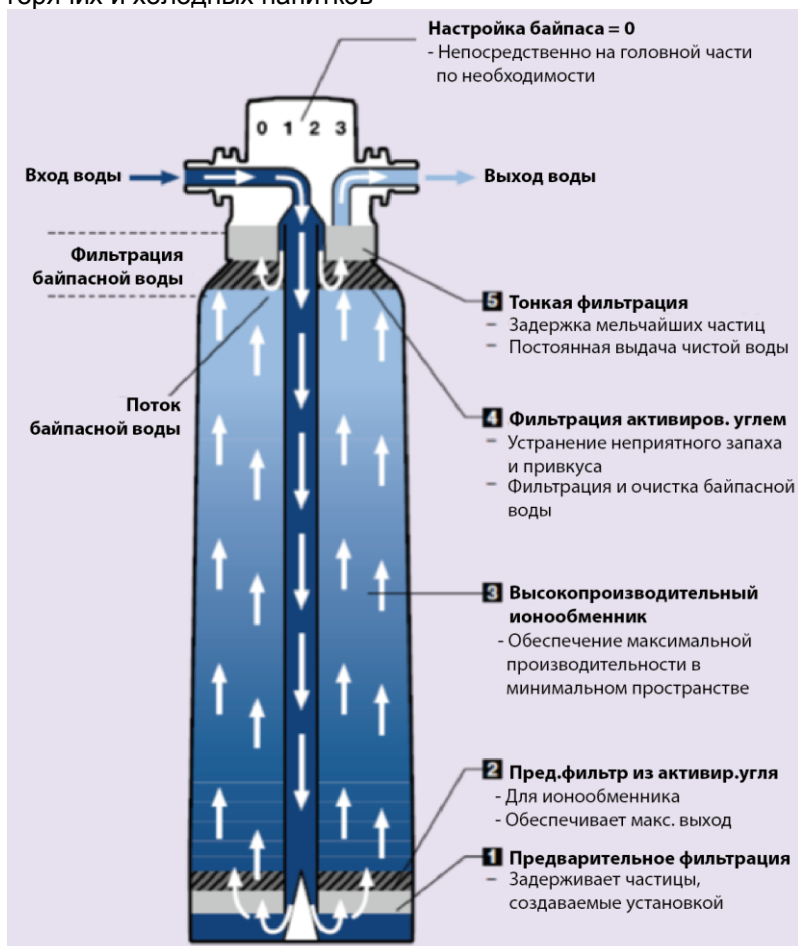
Конфигурация фильтрующего картриджа BWT bestprotect с 5-фазовой фильтрацией
